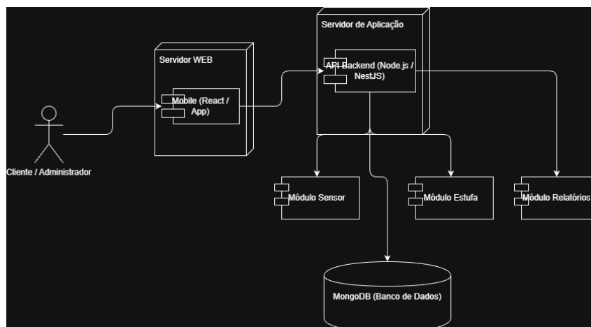
Figura 12: Diagrama de Implantação – Selene
