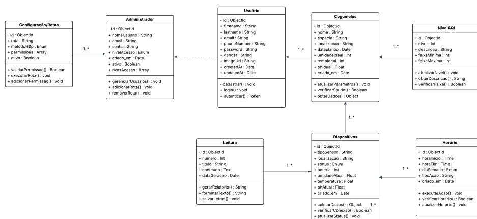
Figura 7: Diagrama de Classes – Selene
